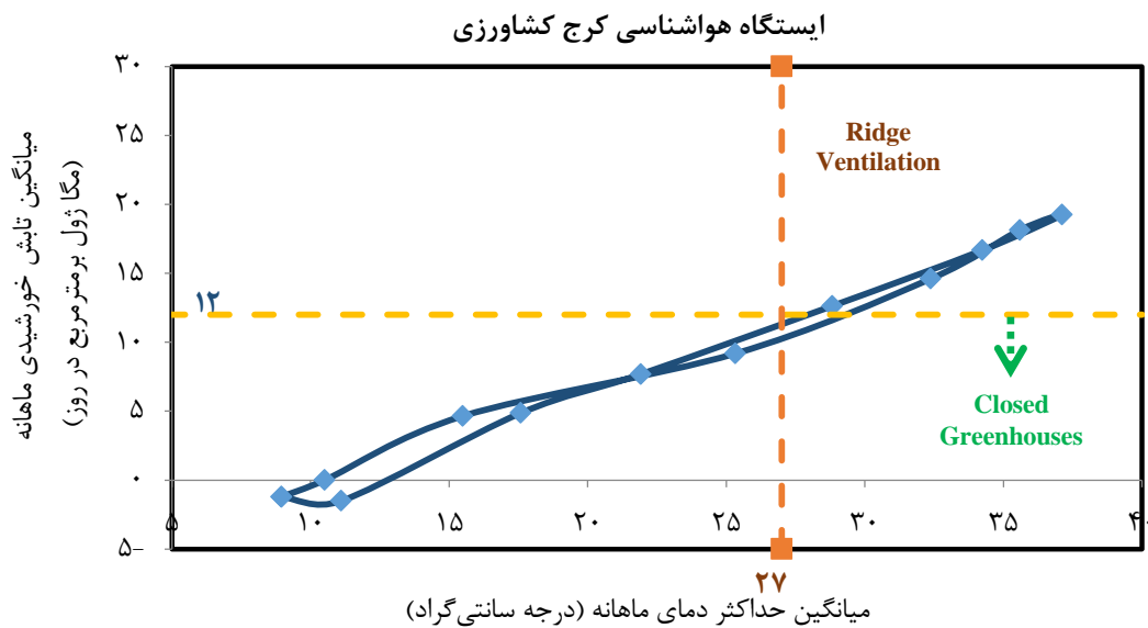
شکل ۲- میانگین دمای حداکثر ماهانه و میانگین تابش خورشیدی ماهانه در ایستگاه هواشناسی کرج
